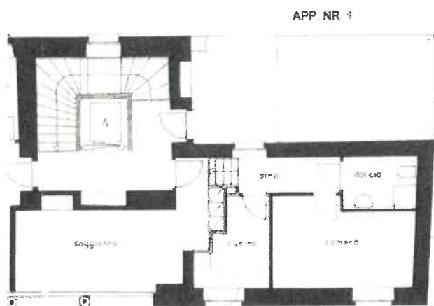
Grundriss
