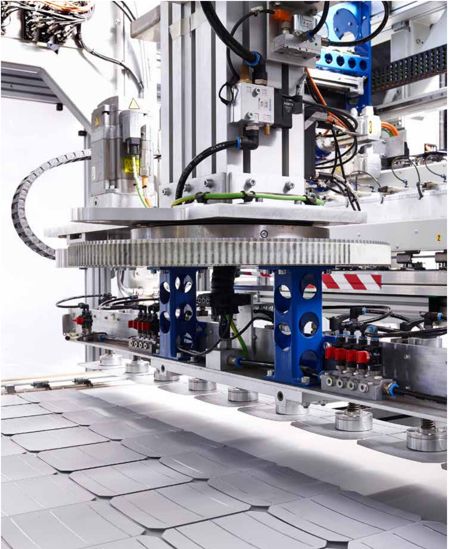
Produktionshalle B: Vollautomatisches Layup von kundenspezifischen PV-Modulen - das Herz einer weltweit einzigartigen Produktionsstrasse
