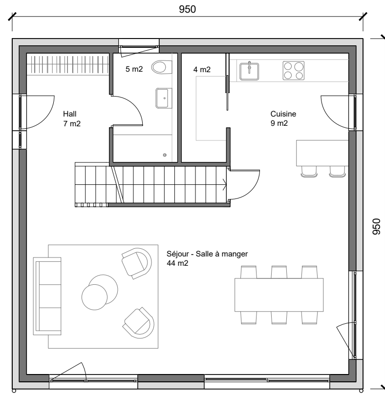
Rez-de-chaussée Villa B
