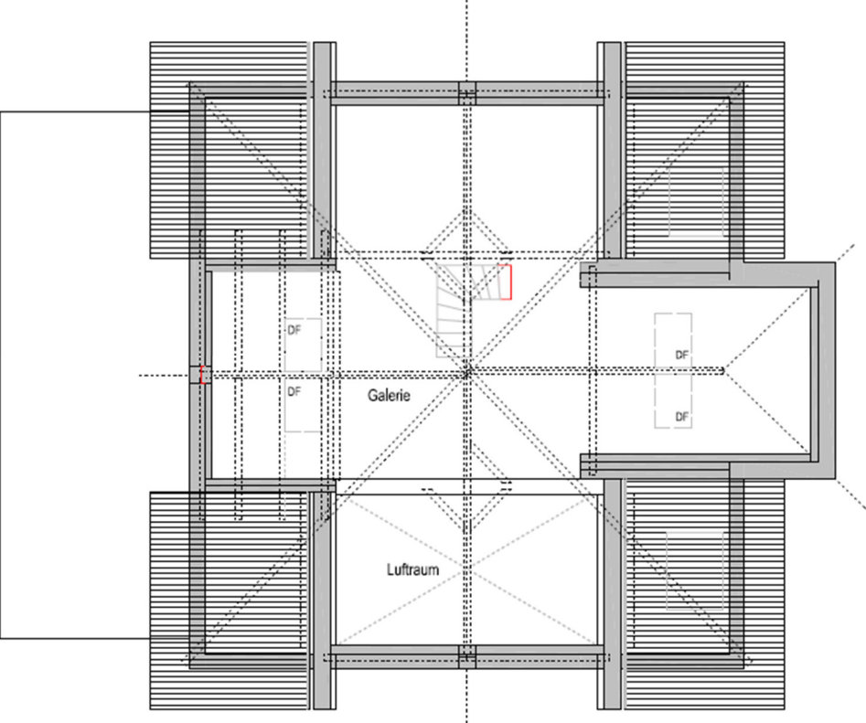
Grundrissplan Galerie
