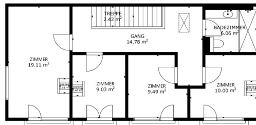
ERDGESCHOSS
