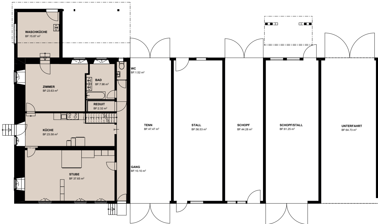
Grundriss Erdgeschoss
