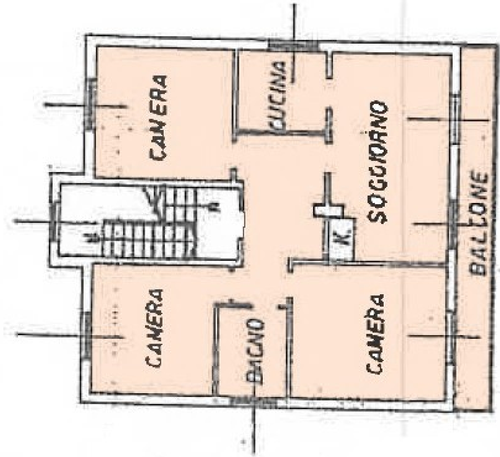
PIANTA PIANO PRIMO h.290
