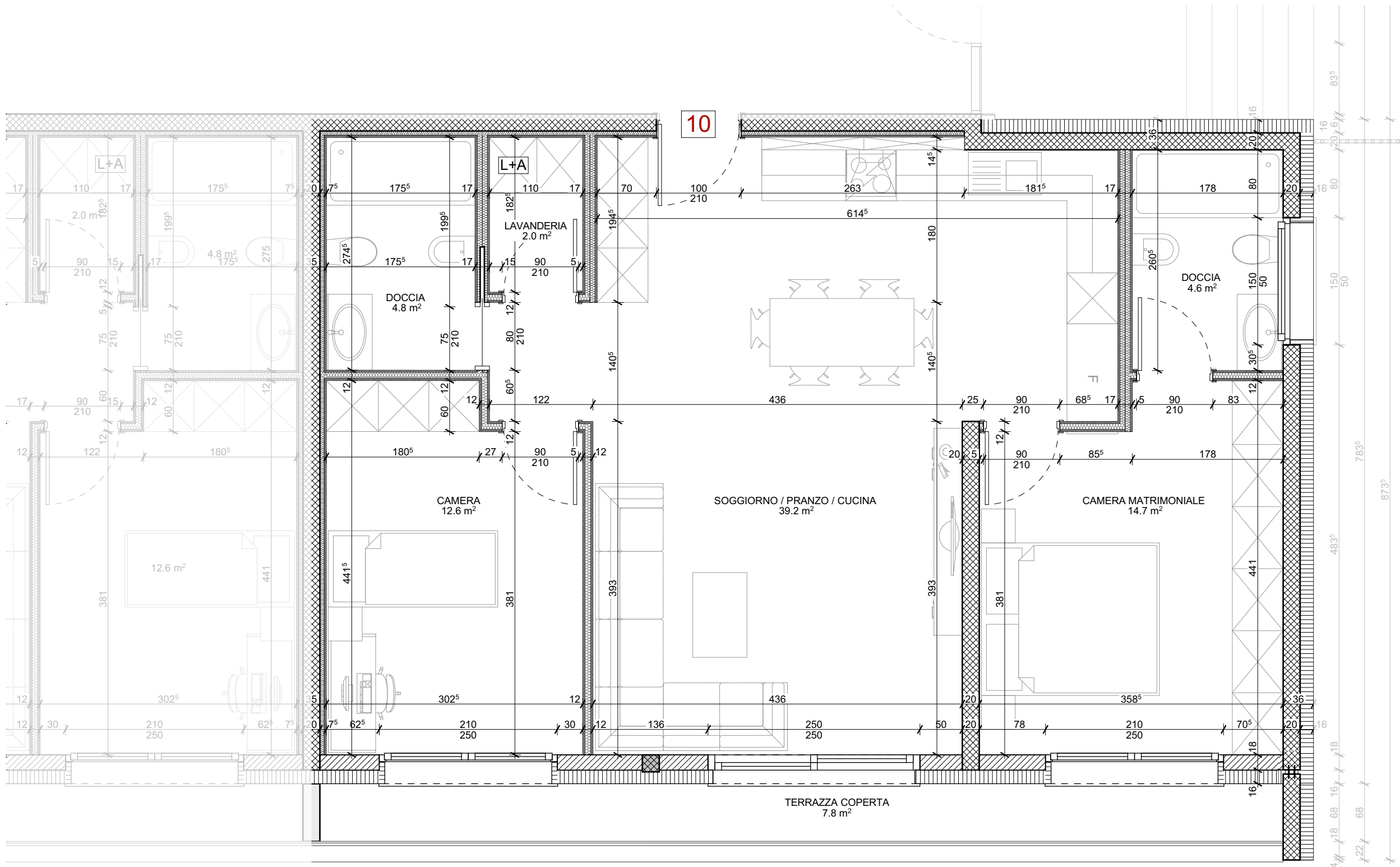
Pianta appartamento
