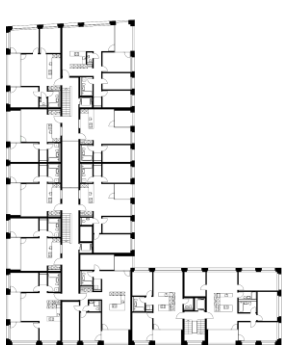
Geschossübersicht
