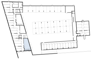
Geschossübersicht
