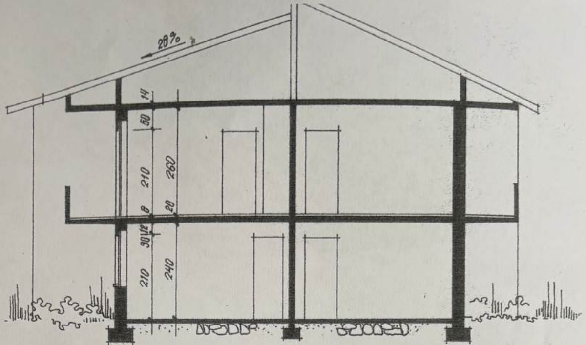
SEZIONE A-A'
