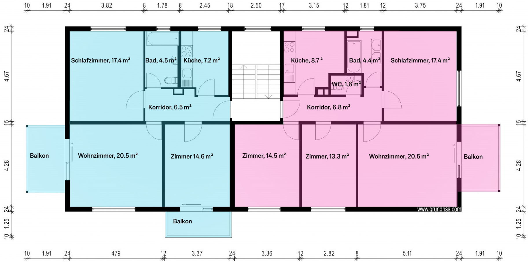
1. u. 2. Obergeschoss
