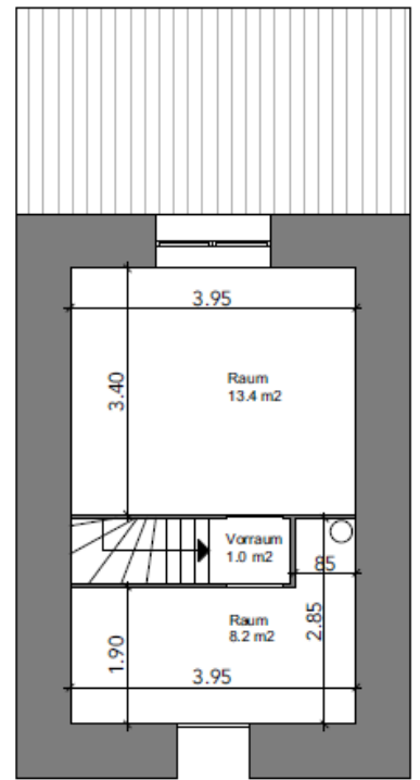
Grundriss 1.Obergeschoss
