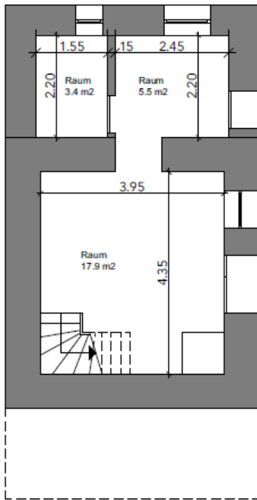
Grundriss Erdgeschoss
