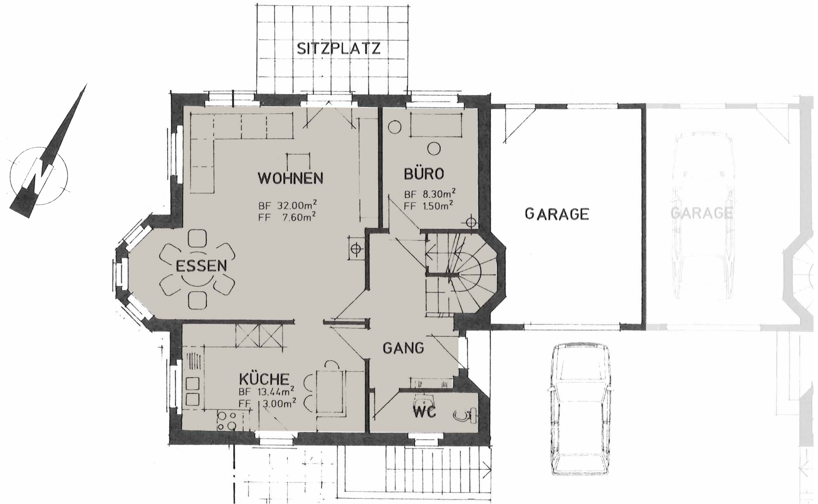
Grundriss Erdgeschoss
