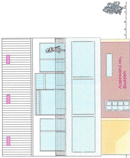
FASSADE SÜD-WEST
