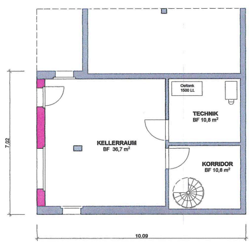
GRUNDRISS UG
