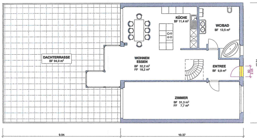
GRUNDRISS OG
