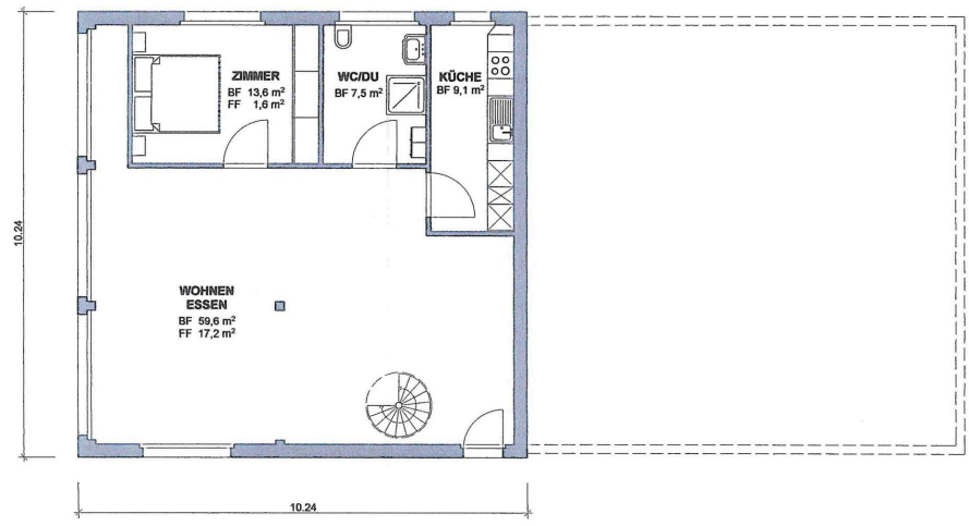
GRUNDRISS EG
