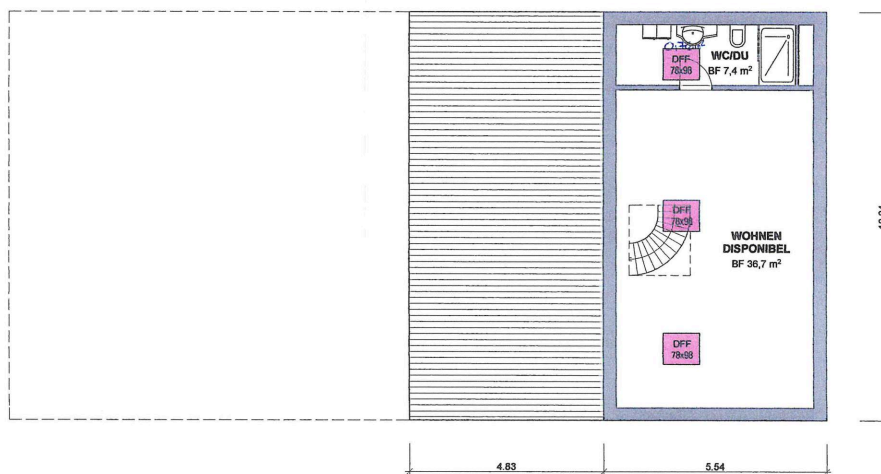
GRUNDRISS DG
