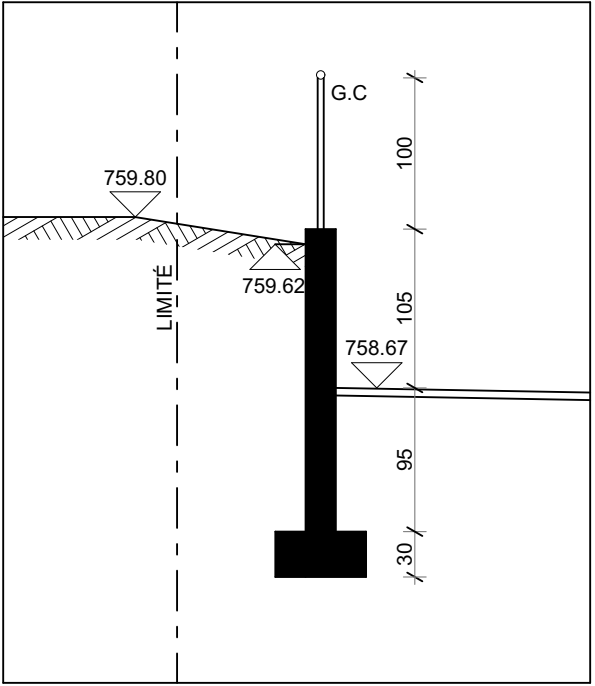
COUPÉ 2-2
