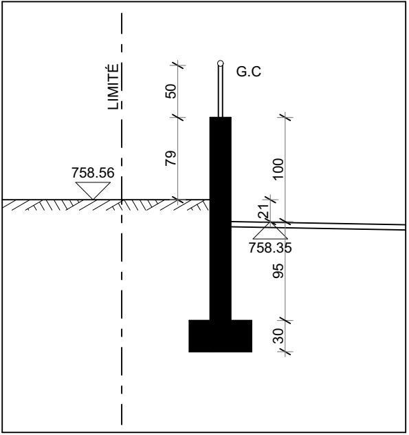
COUPÉ 1-1
