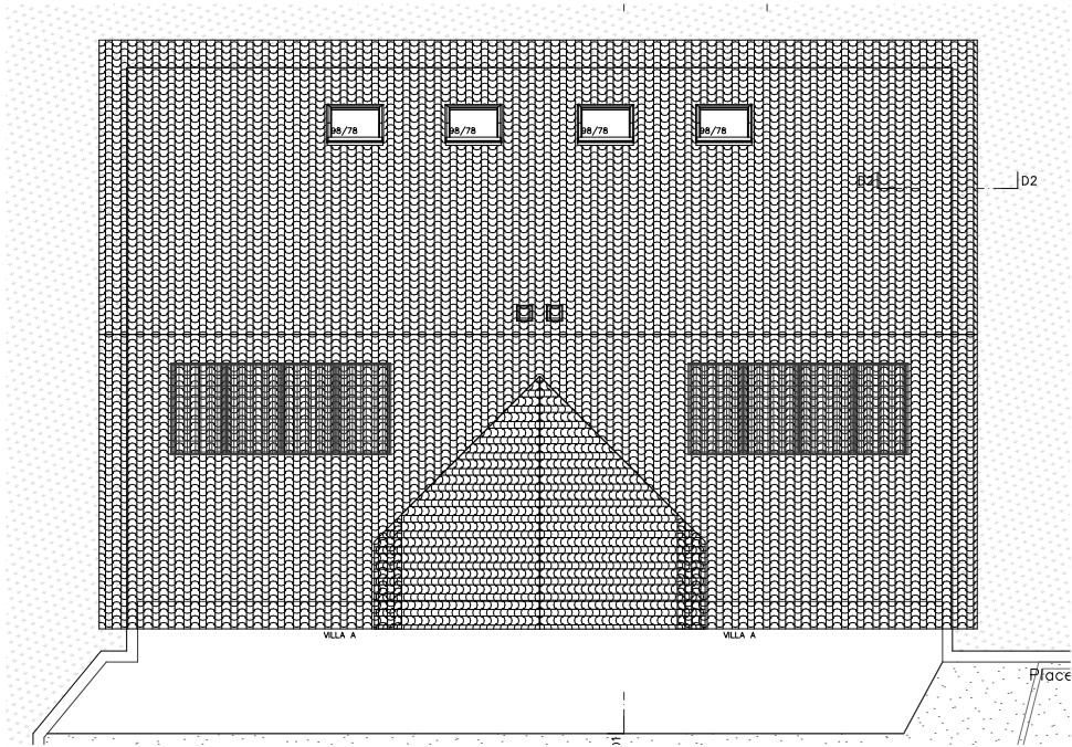
PLAN COUVERTURE
