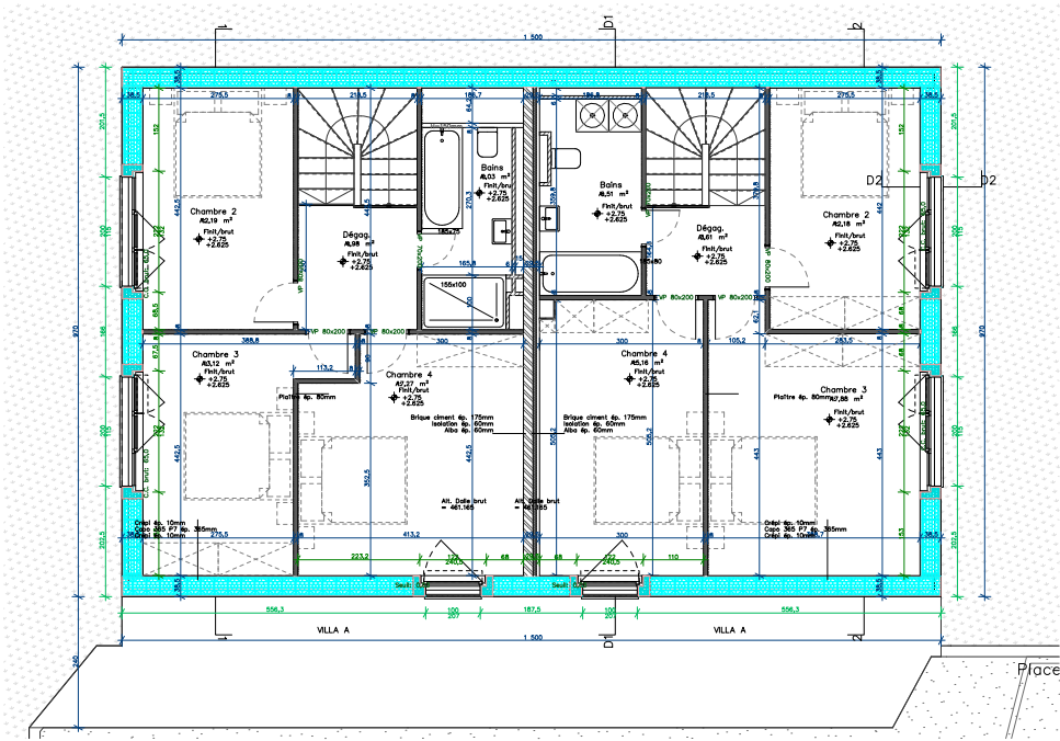
PLAN ETAGE
