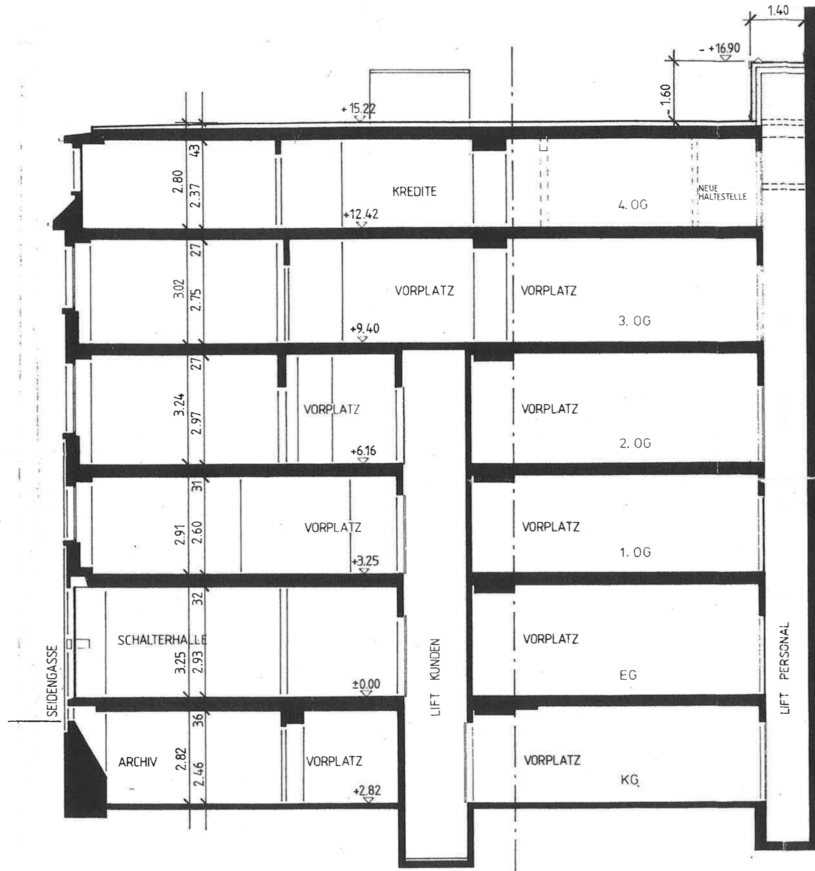
SCHNITT A-A
