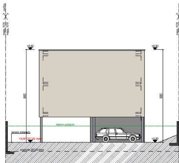
PROSPETTO OVEST
