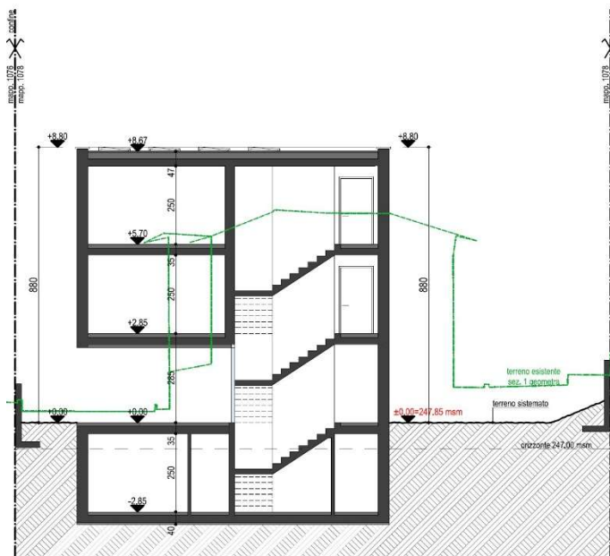
SEZIONE A-A
