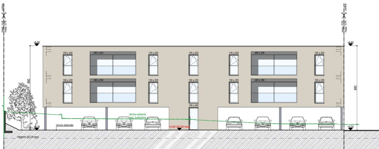
PROSPETTO SUD
