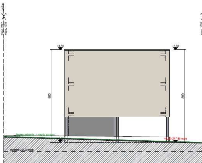
PROSPETTO EST
