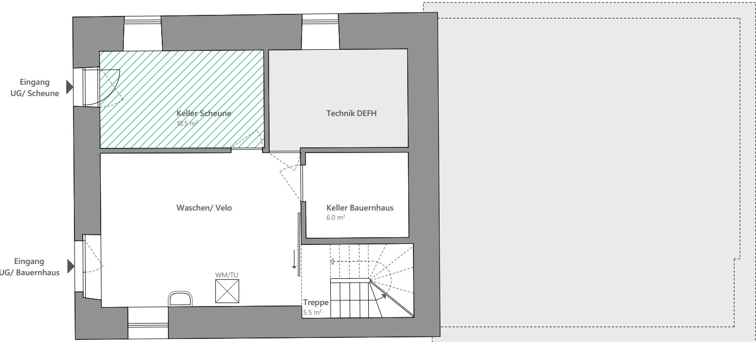
Untergeschoss
