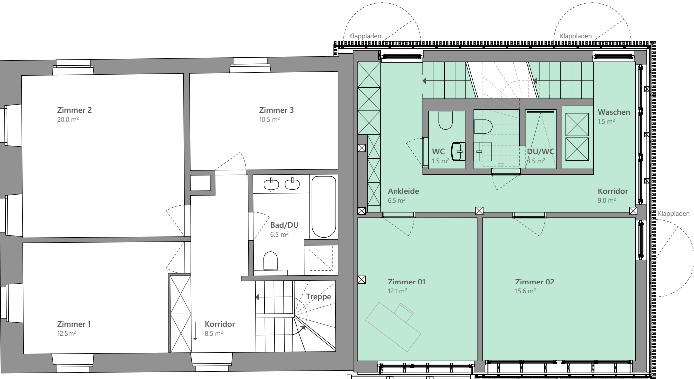
1. Obergeschoss
