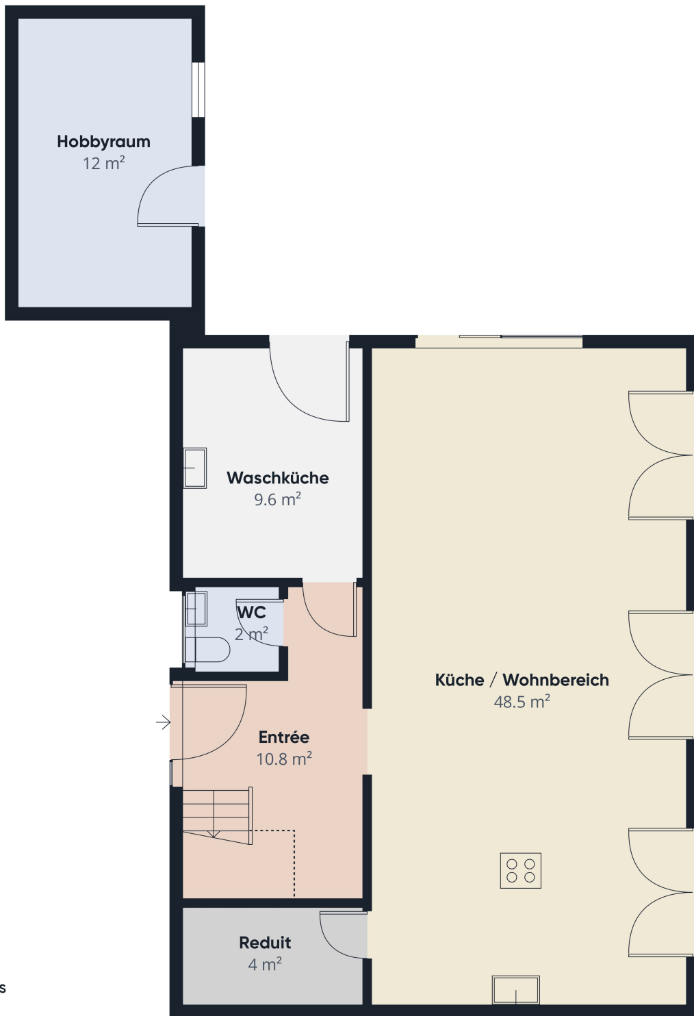
Etage 0
