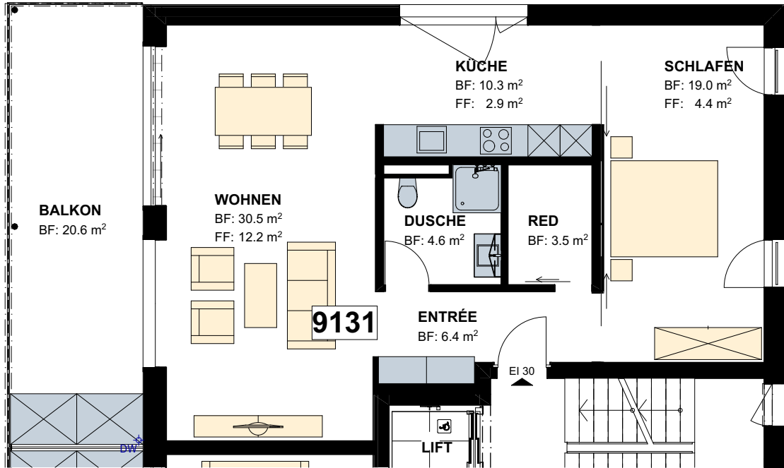
3. Obergeschoss Nord
