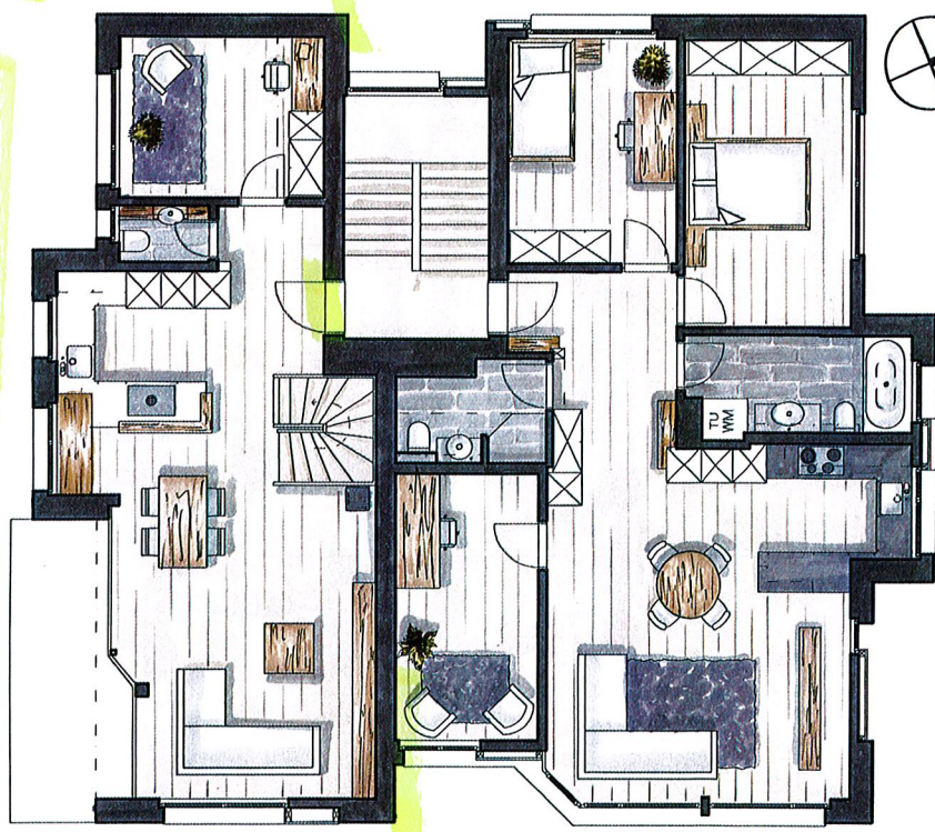
2. OG, 4.5 - ZIMMER MAISONETTE - WOHNUNG, 114 m 2
