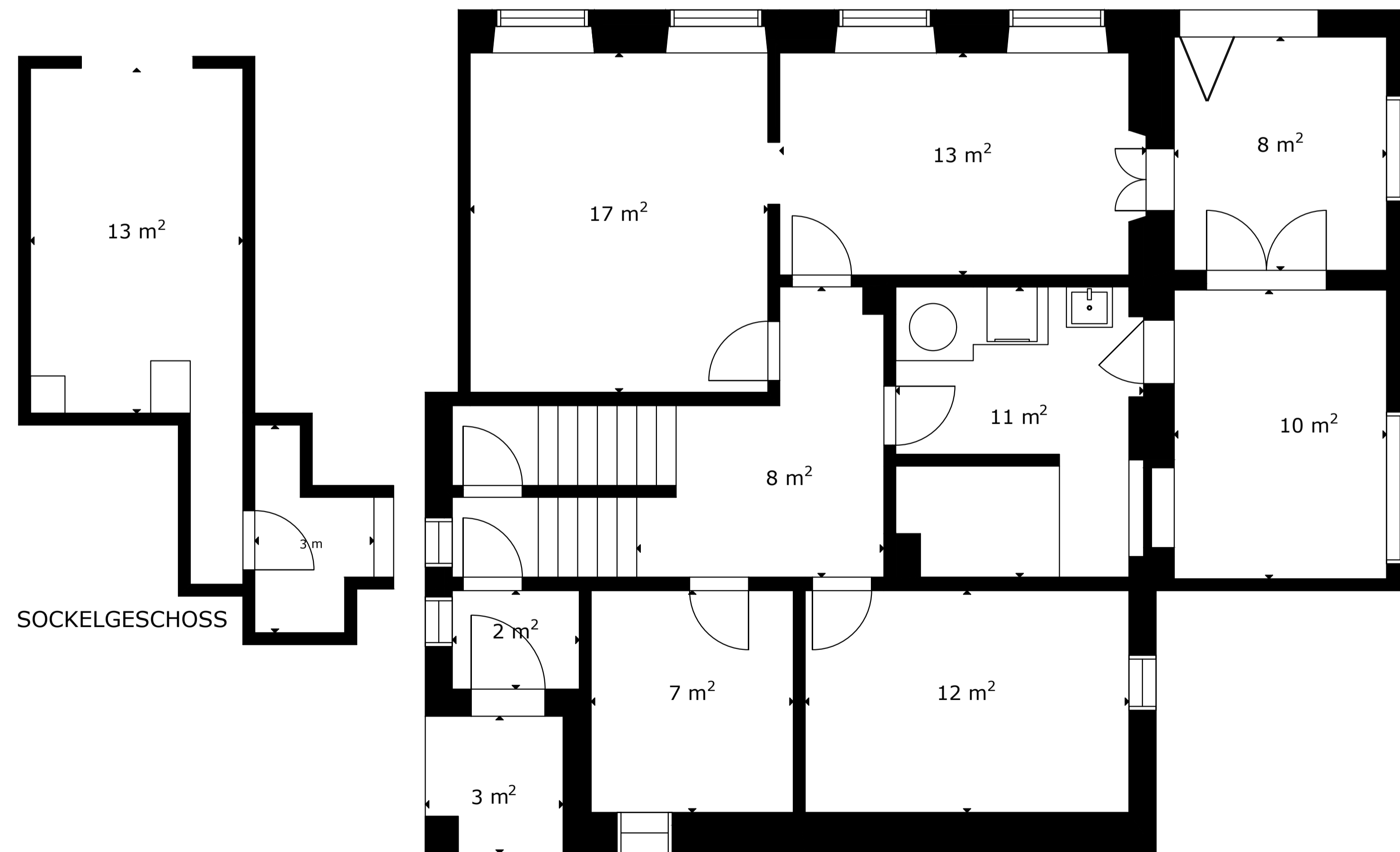
SOCKELGESCHOSS
