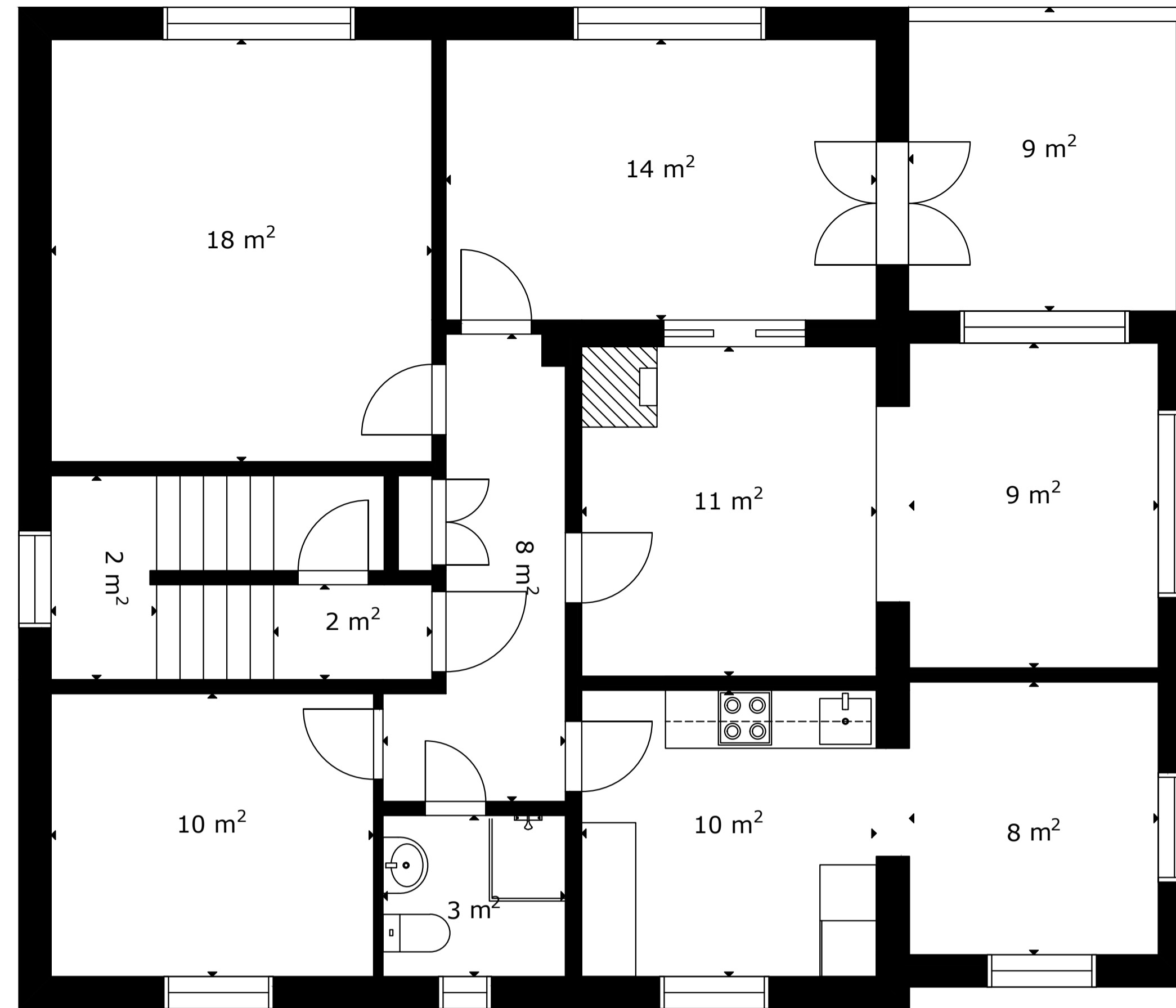
2.OBERGESCHOSS
