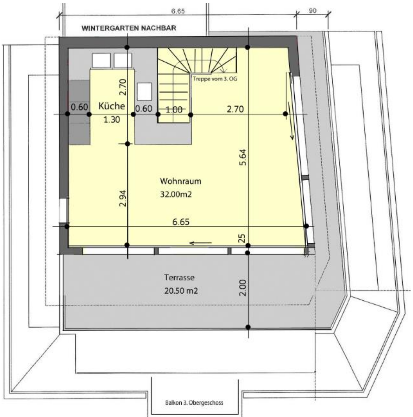
Grundriss Dachgeschoss
