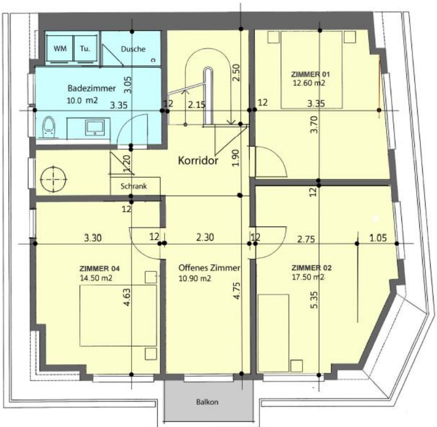
Grundriss 3. Obergeschoss
