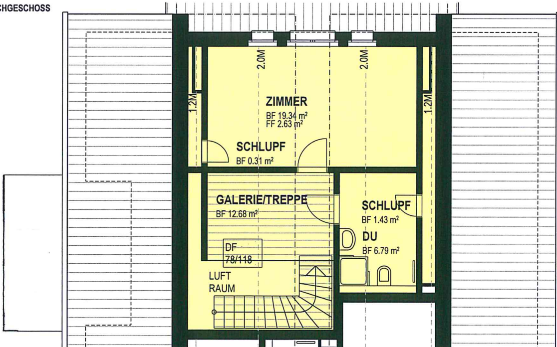
GRUNDRISS DACHGESCHOSS
