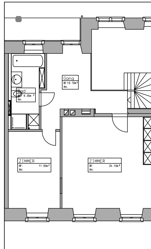
2. Obergeschoss
