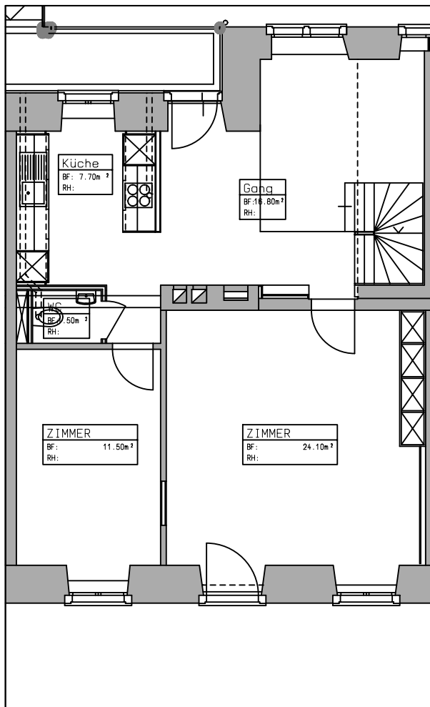
1. Obergeschoss
