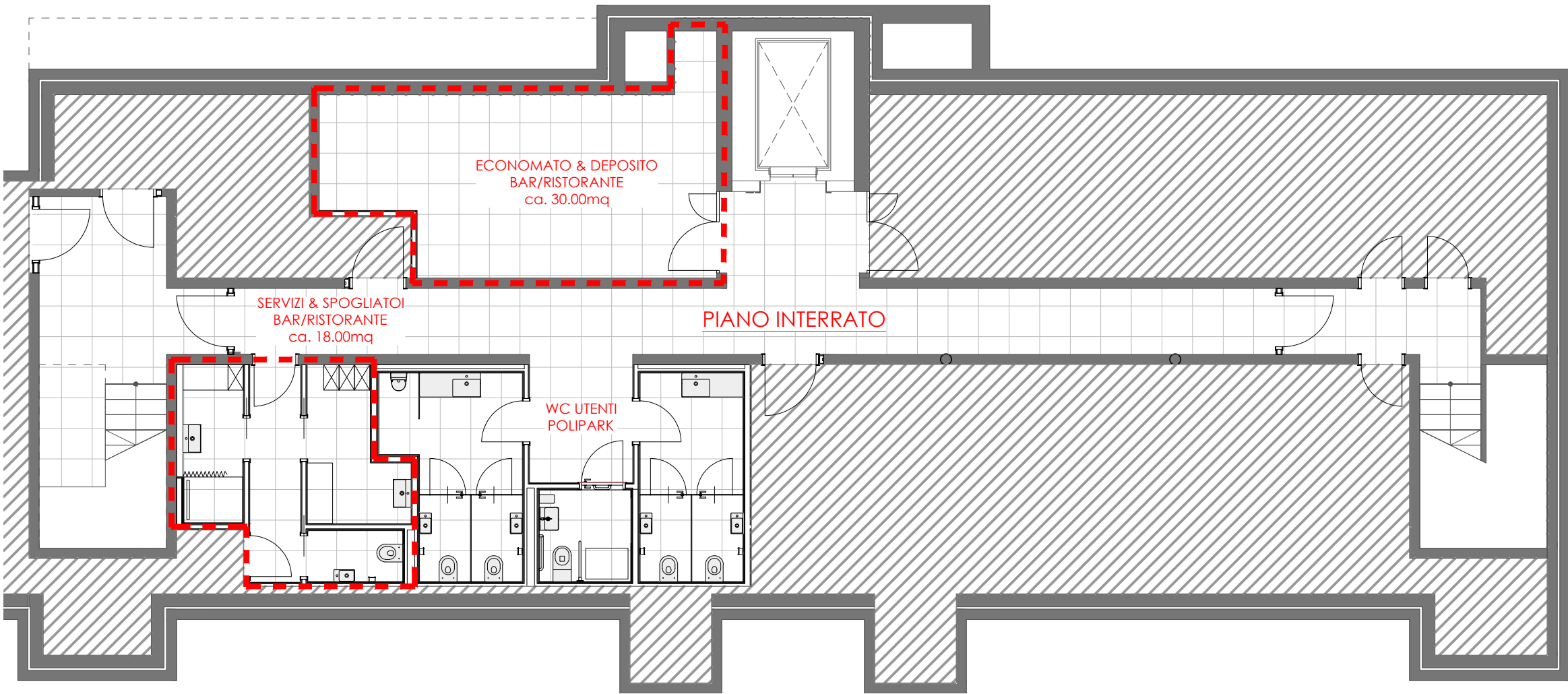
PIANTA PIANO INTERRATO BLOCCO B
