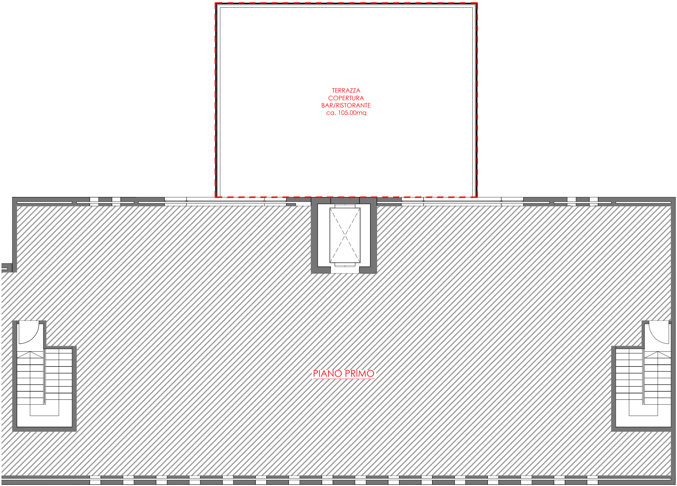
PIANTA PIANO PRIMO BLOCCHI B e H
