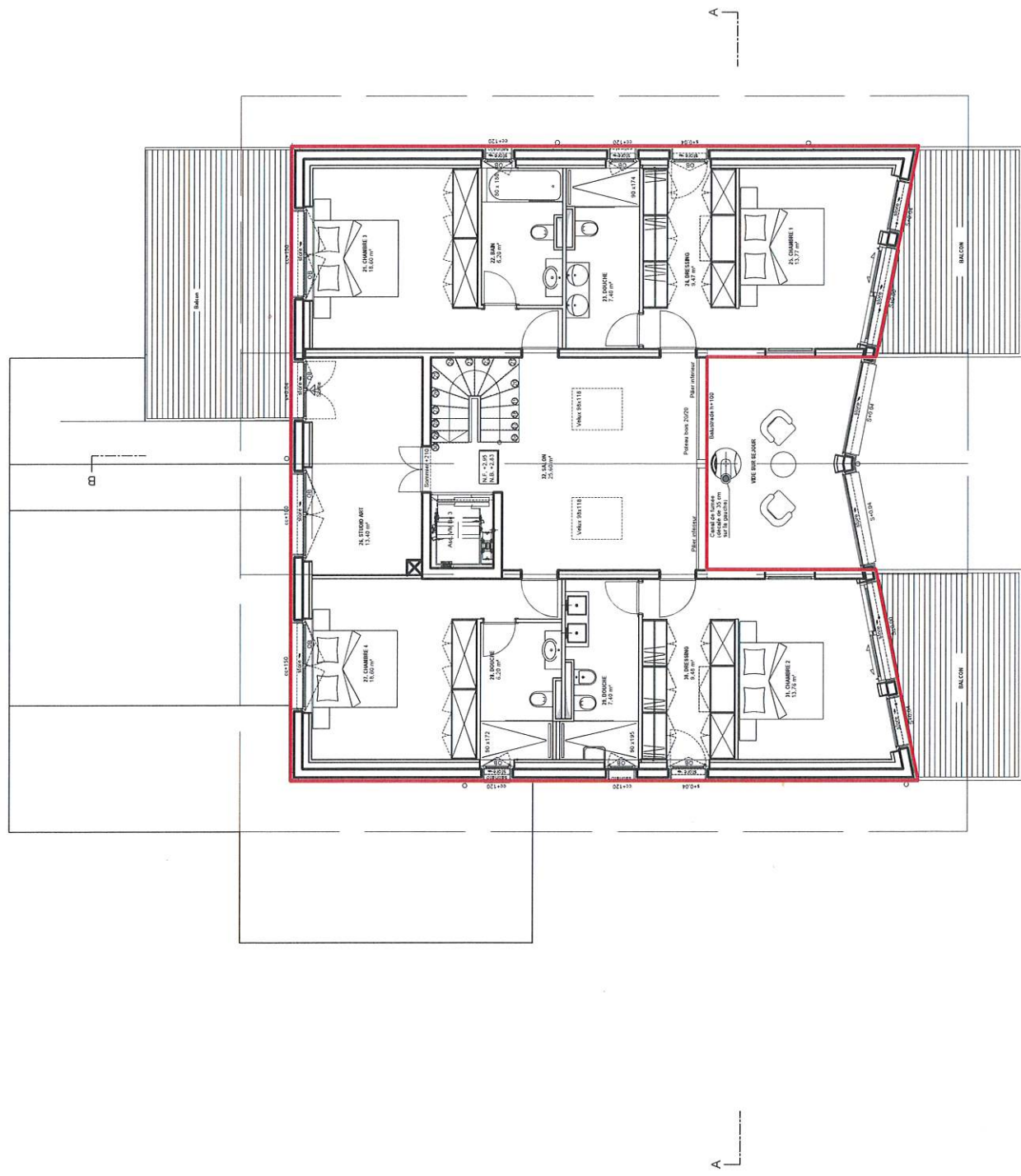
plan de l'étage surface chauffée = 193m2 surface 1/2 balcons = 26m2
