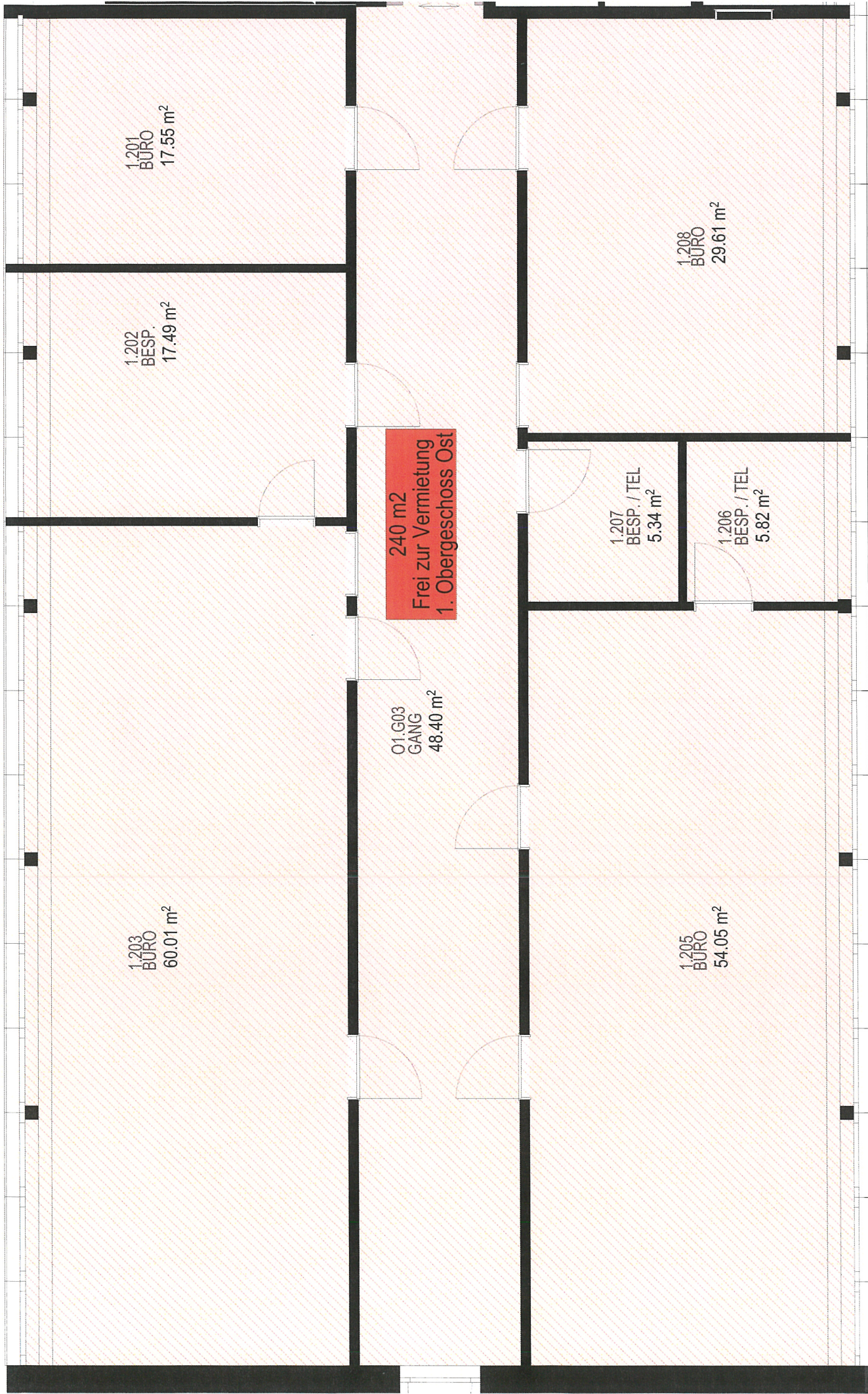
Mietflächen 1. OBERGESCHOSS Mstb. 1:50 1. OG Ost
