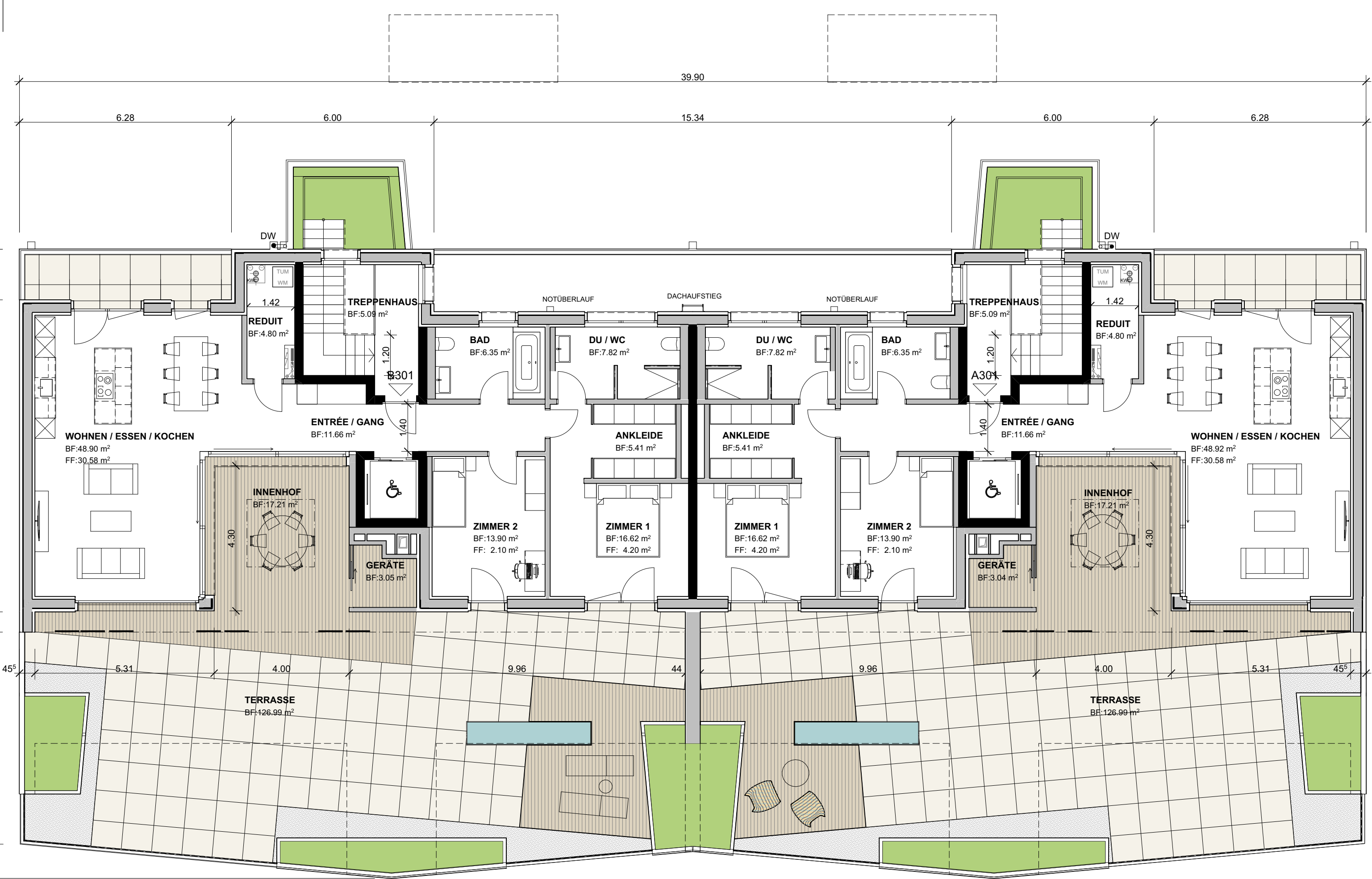
3. OBERGESCHOSS
