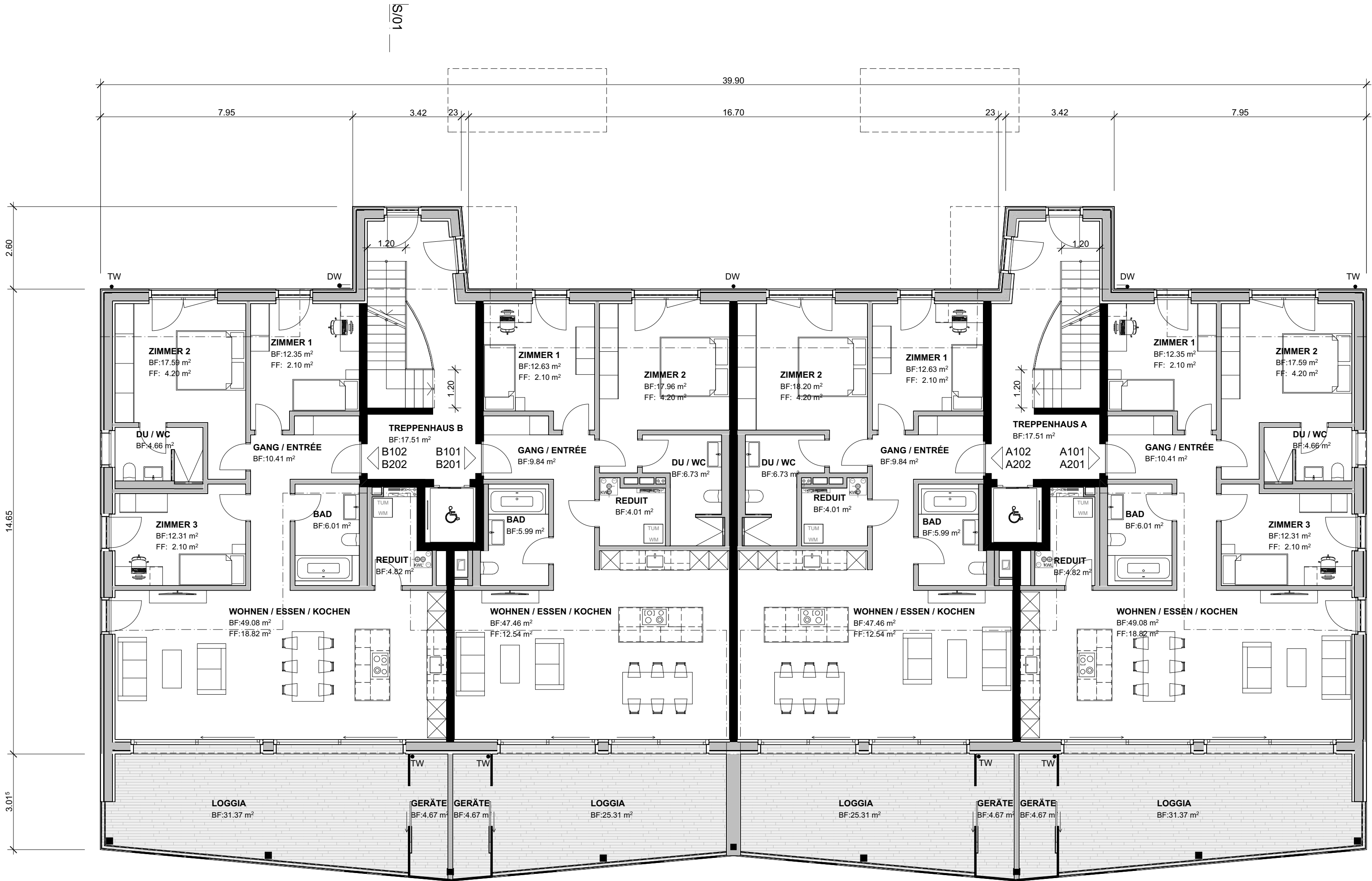
1. & 2. OBERGESCHOSS
