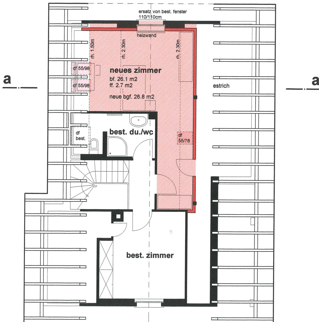
grundriss dachgeschoss
