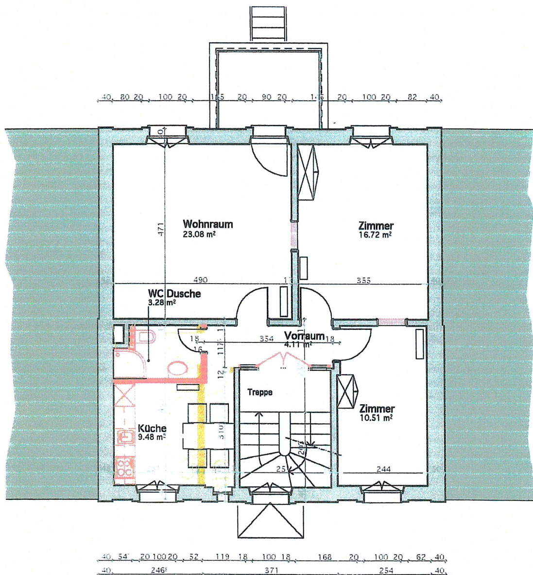
1. Obergeschoss
