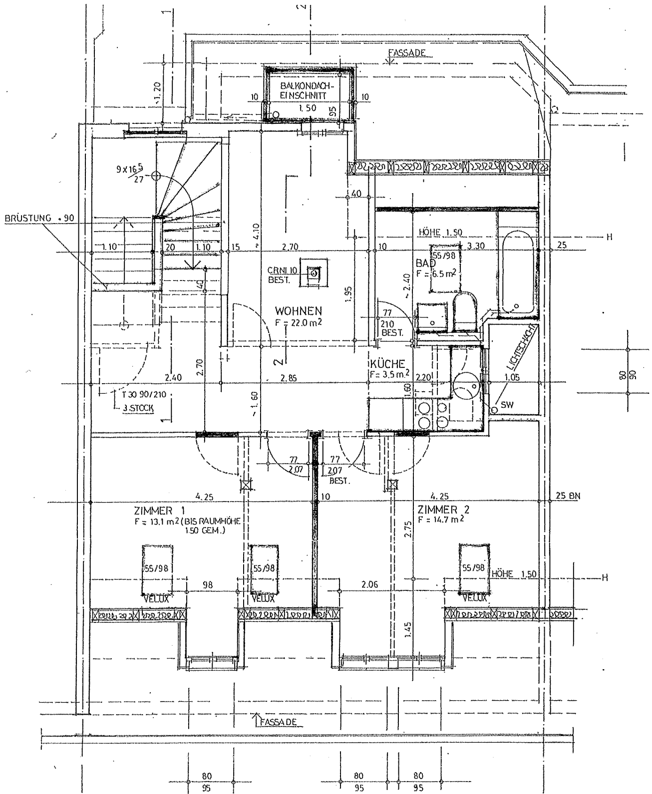
GRUNDRISS DACHGESCHOSS MST. 1 : 50
