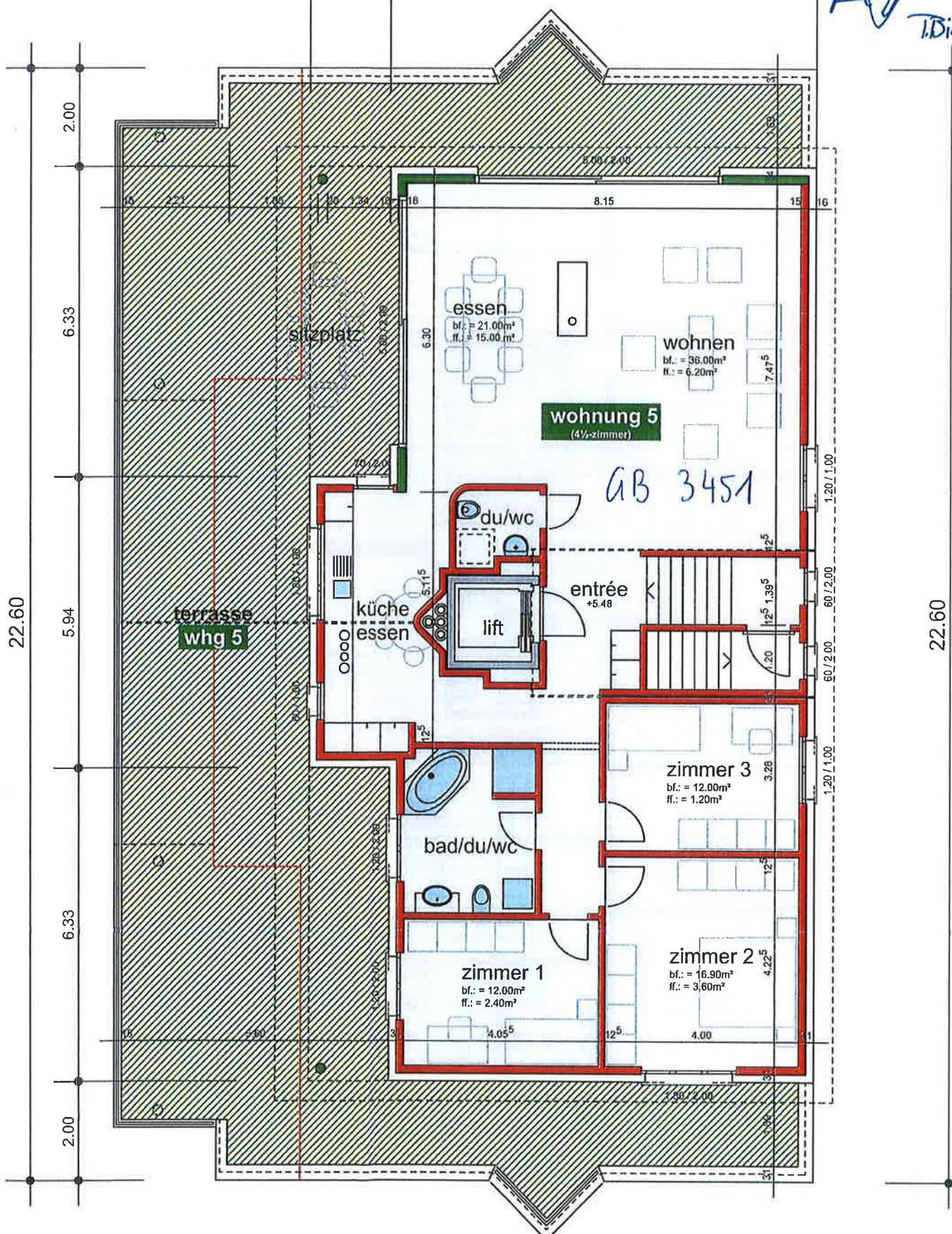
attikageschoss sonnenfeldweg 8
