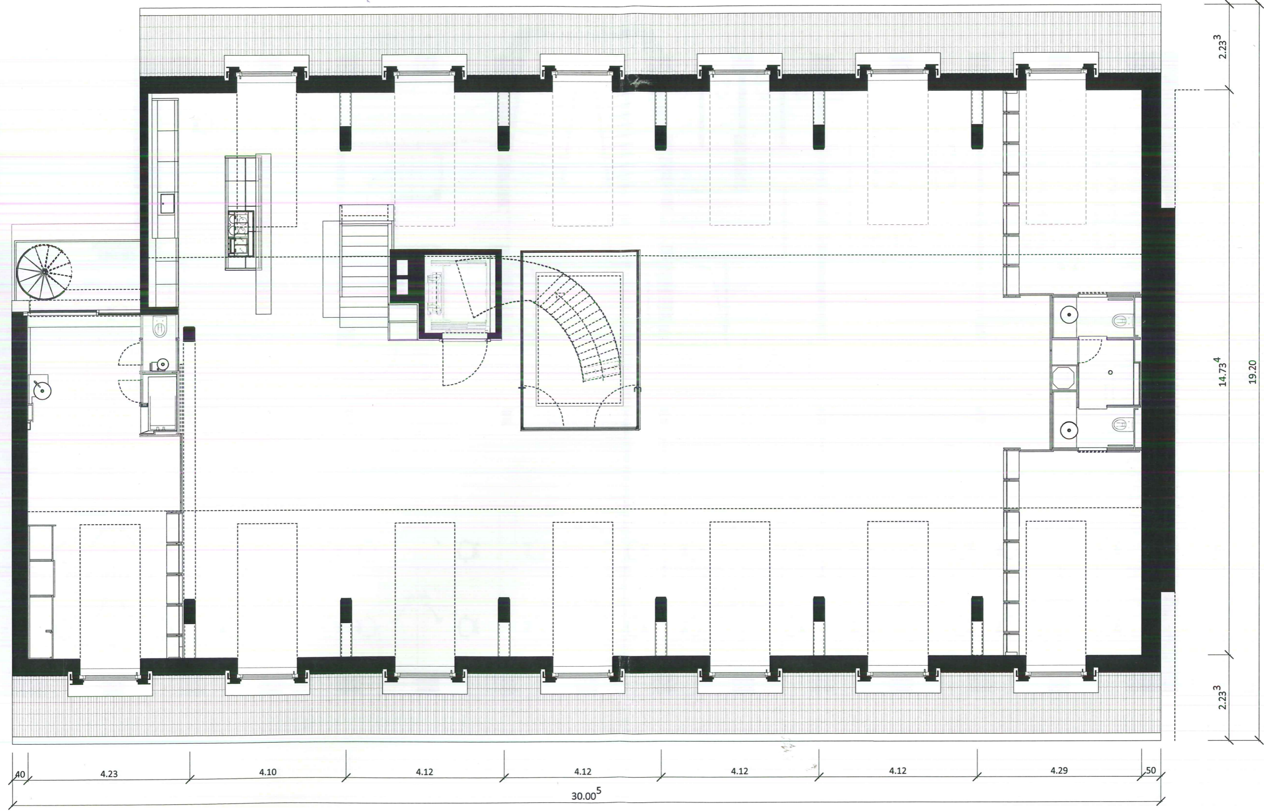
Grundriss Dachgeschoss Bäckerstrasse 40 / 8004 Zürich
