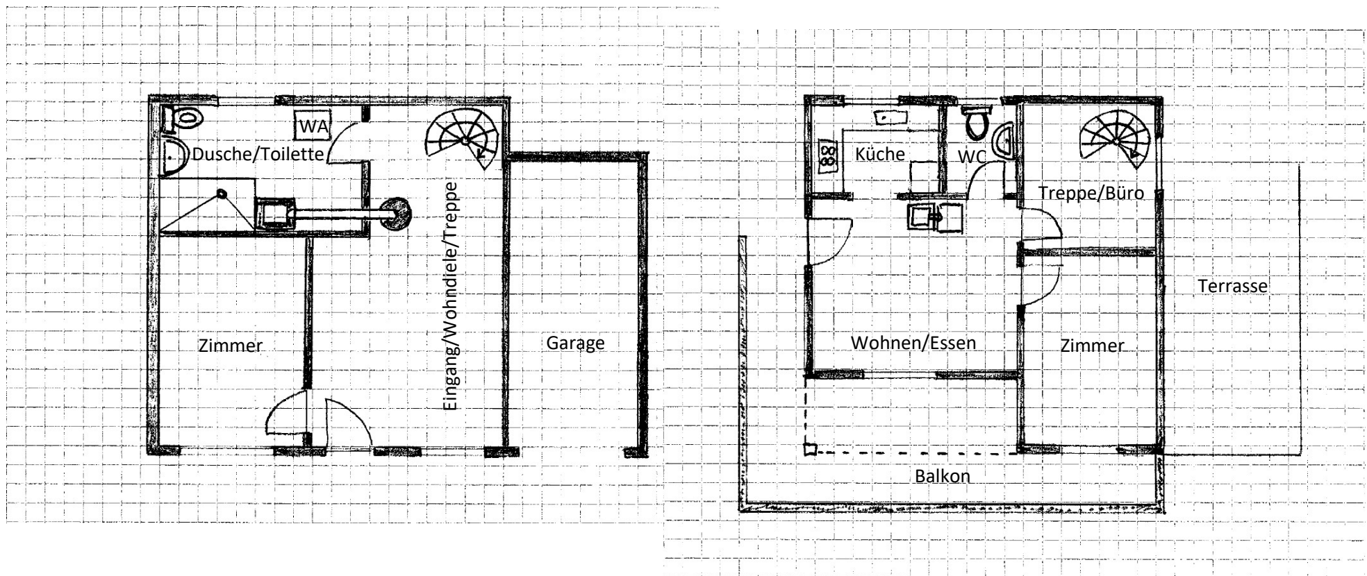
ERDGESCHOSS
