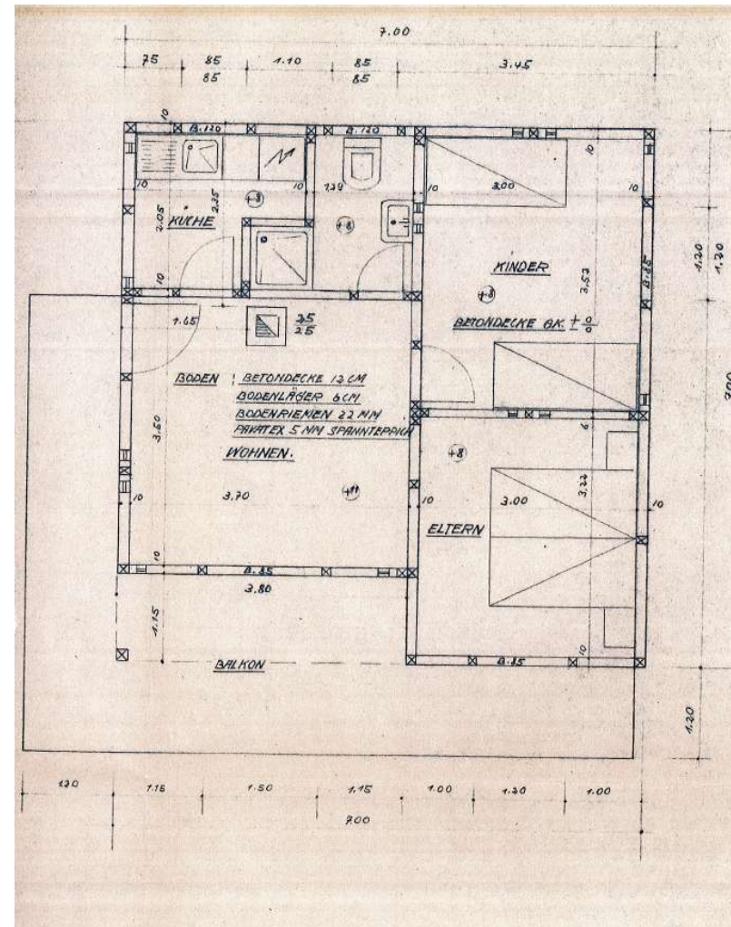
OBERGESCHOSS
