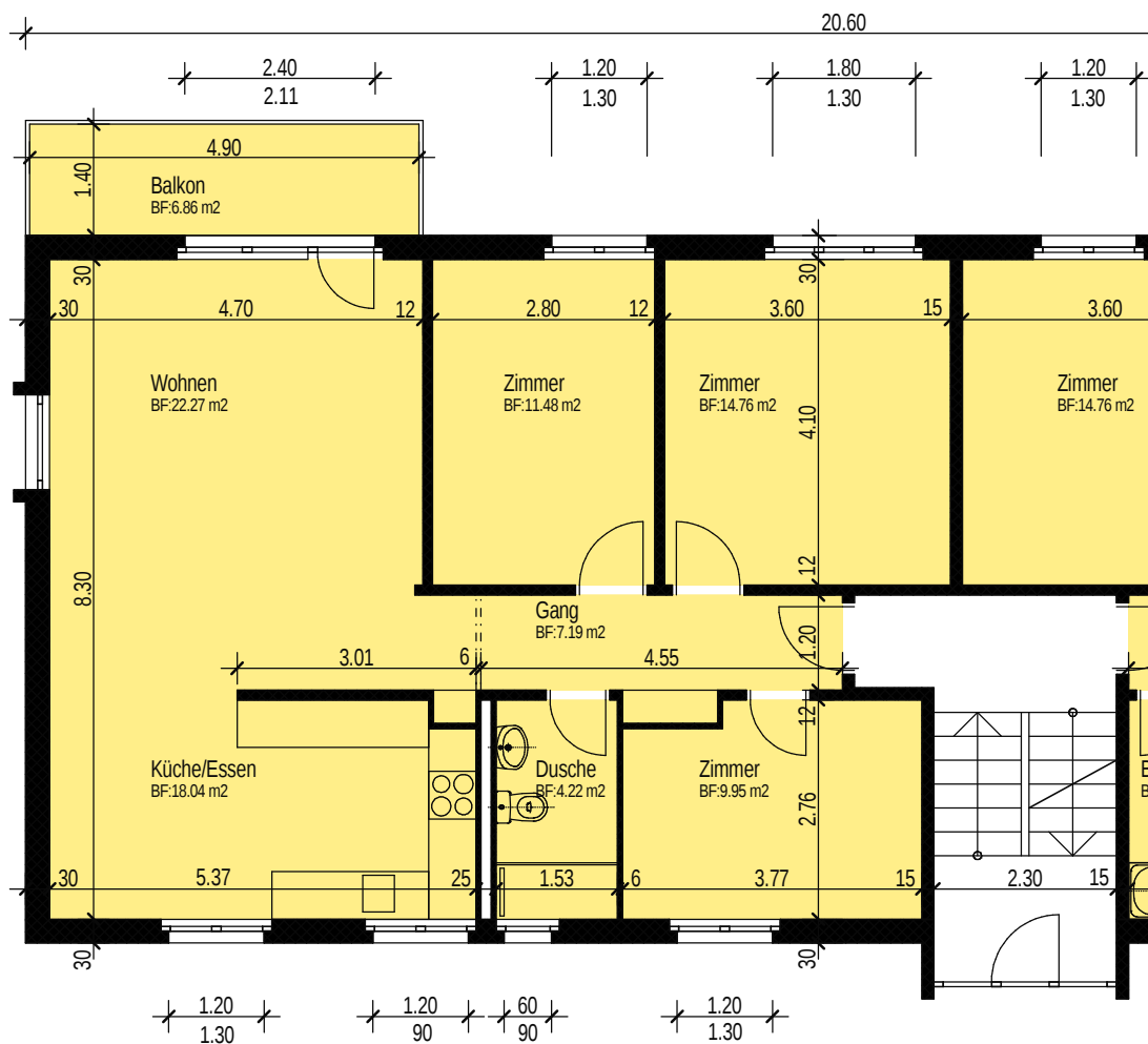
Grundriss
