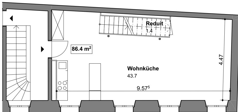
2. Obergeschoss
