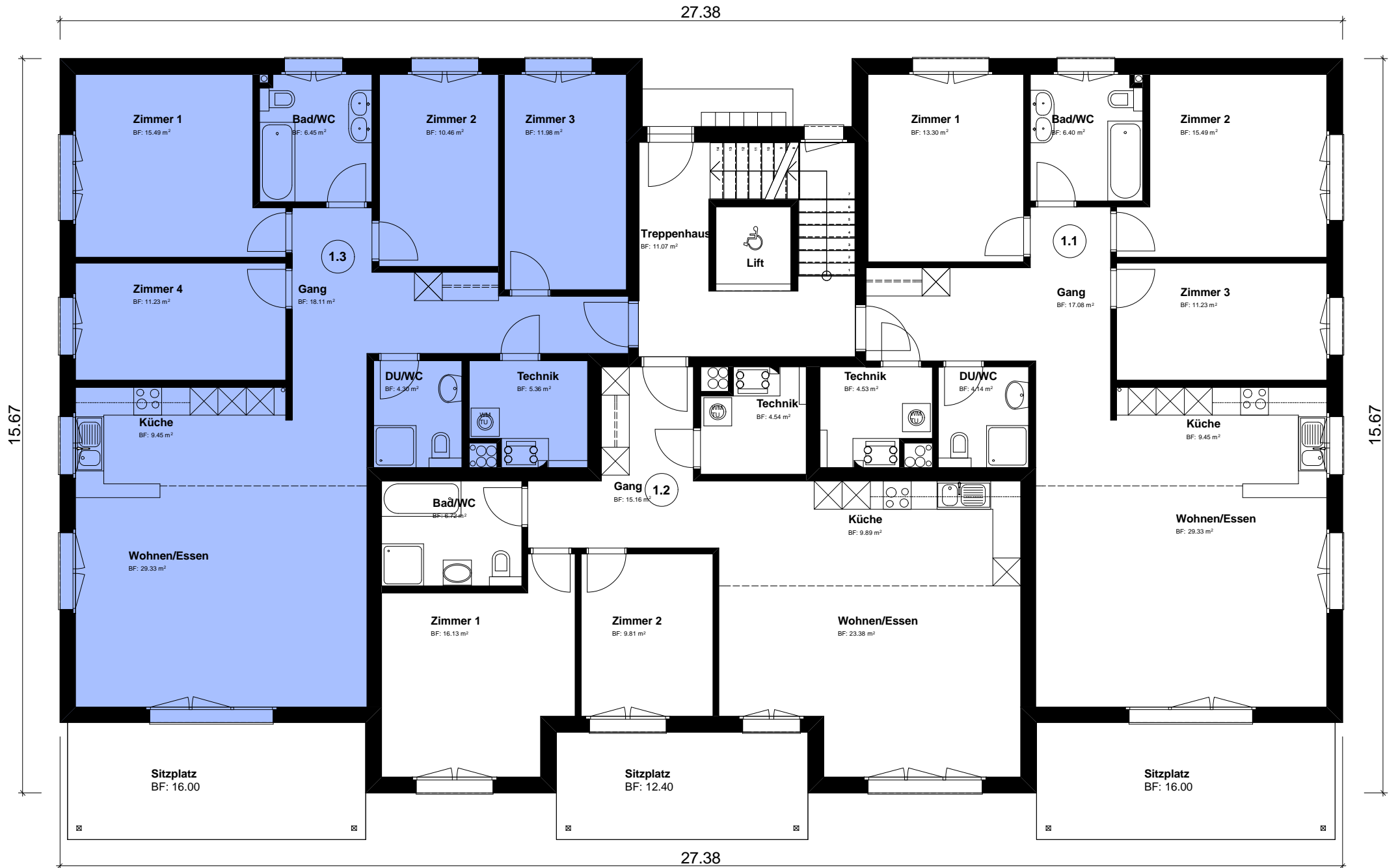
ERDGESCHOSS HAUS A/B/C/E/F
