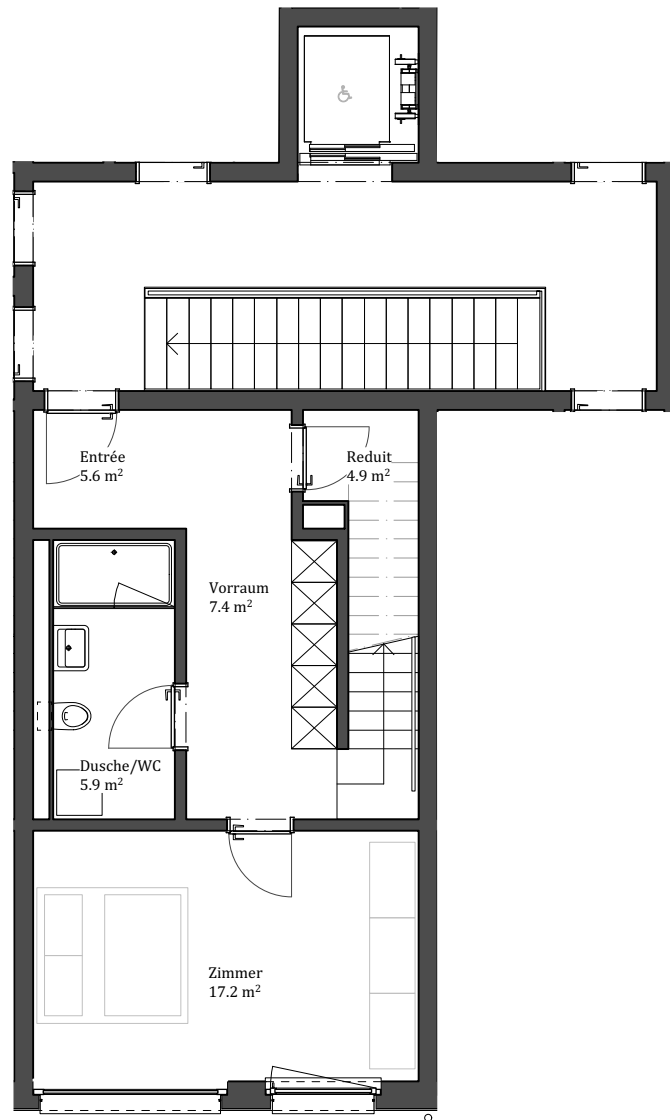
Wohnung 1.1 Obergeschoss
