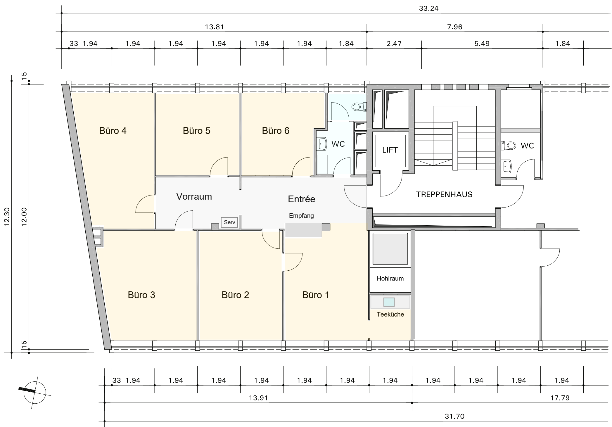
3. Obergeschoss (Nord) 1 : 100
