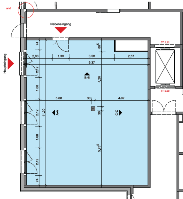
Grundriss
