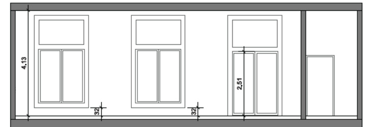
Ansicht A-A
