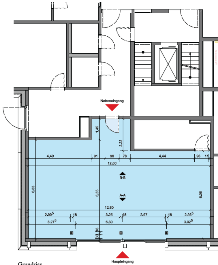
Grundriss
