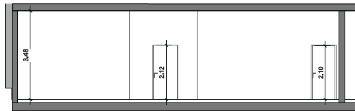
Ansicht A-A
