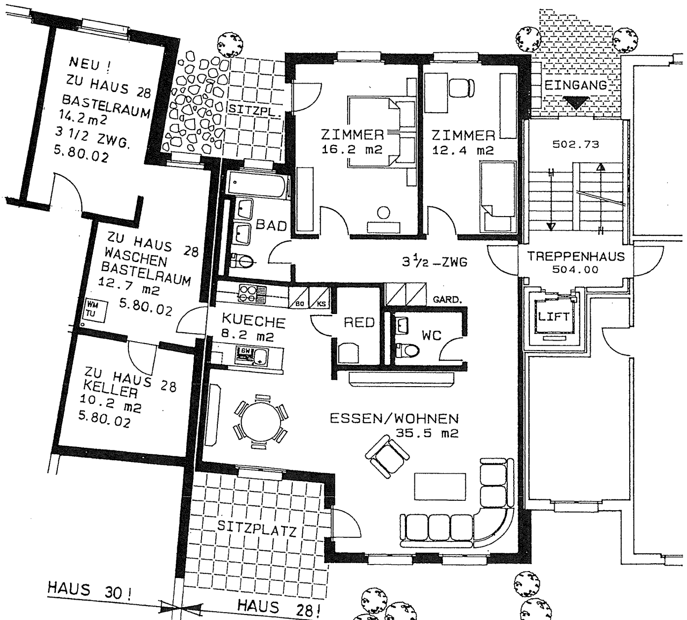
GRUNDRISS MST. 1: 100
