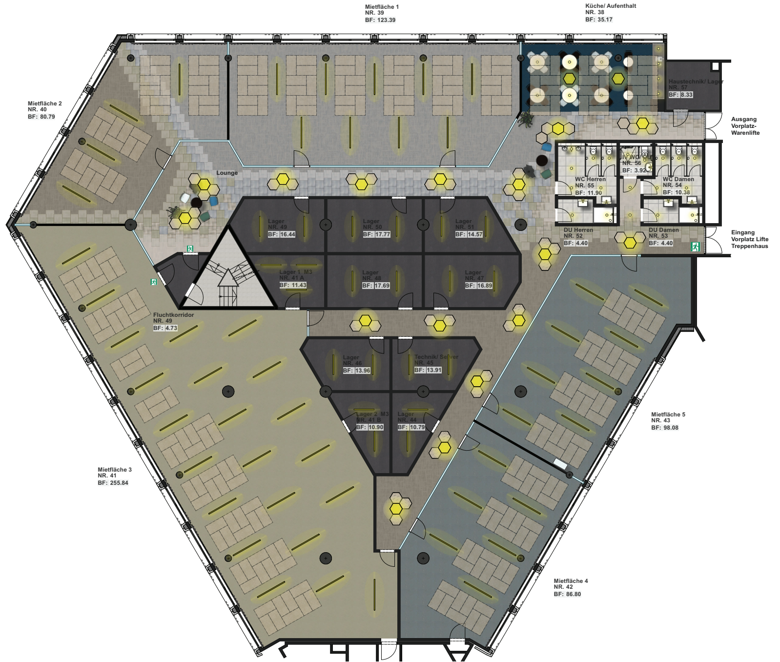
3. Obergeschoss Industriestrasse 5/7
