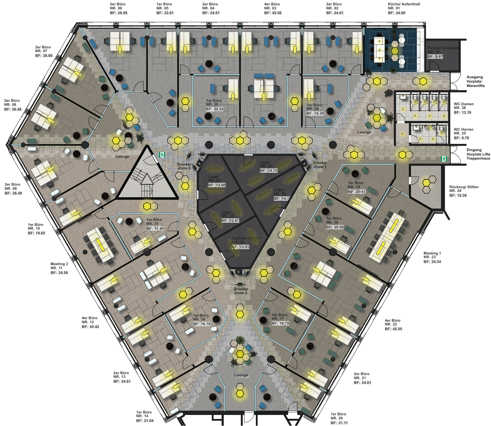
2. Obergeschoss Industriestrasse 5/7
