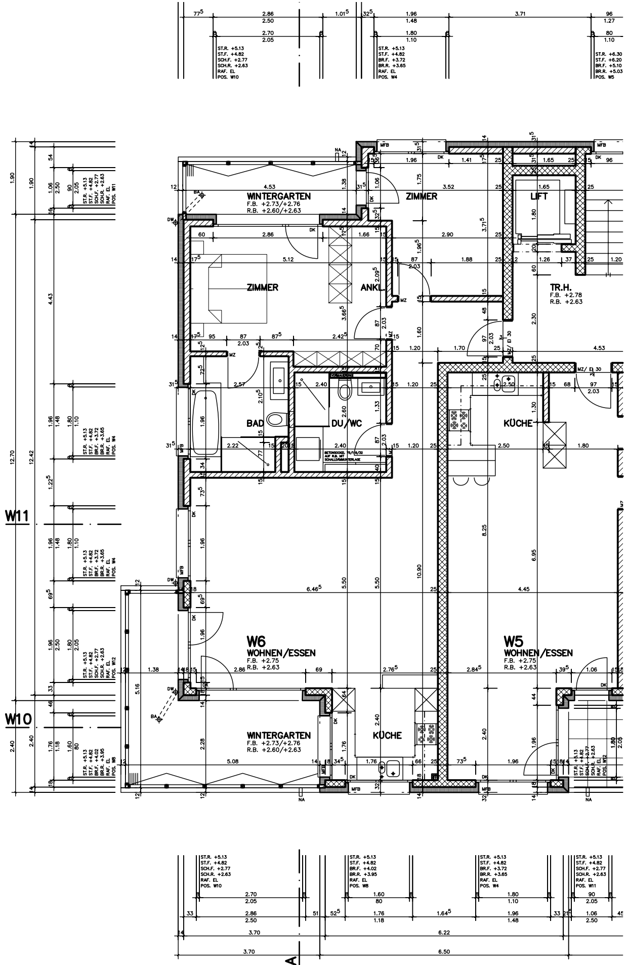
1. OBERGESCHOSS WOHNUNG W6 1:100
