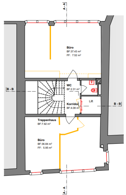
2. OBERGESCHOSS 1:100
