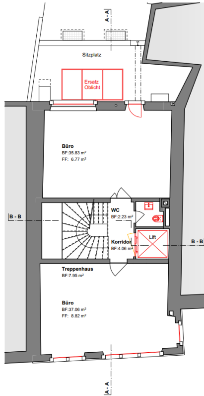
1. OBERGESCHOSS 1:100
