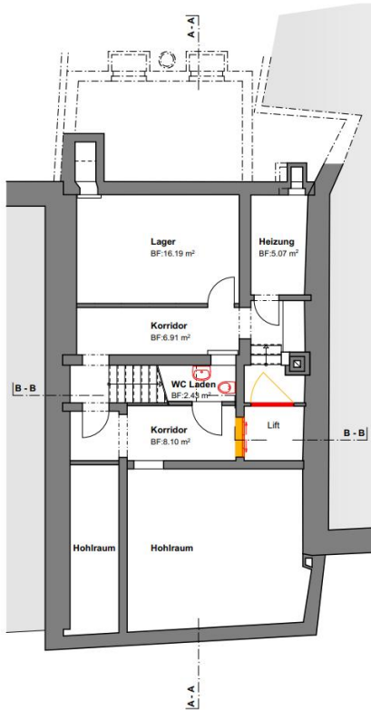
UNTERGESCHOSS 1:100
