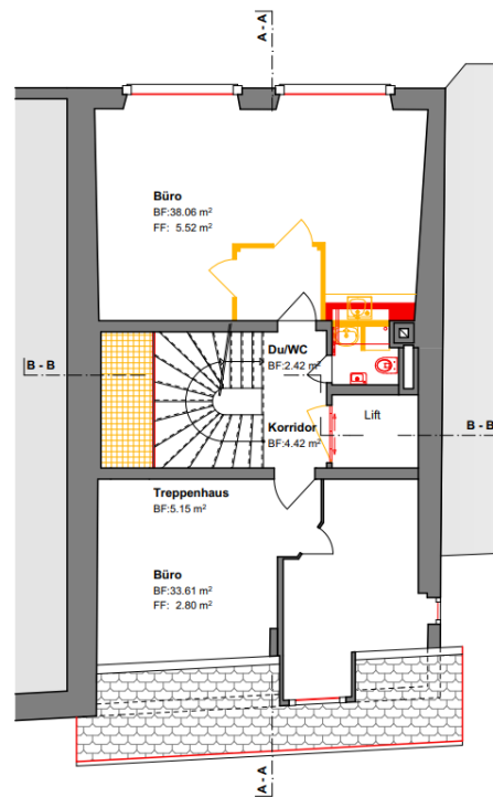
DACHGESCHOSS 1:100
