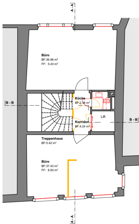
3. OBERGESCHOSS 1:100
