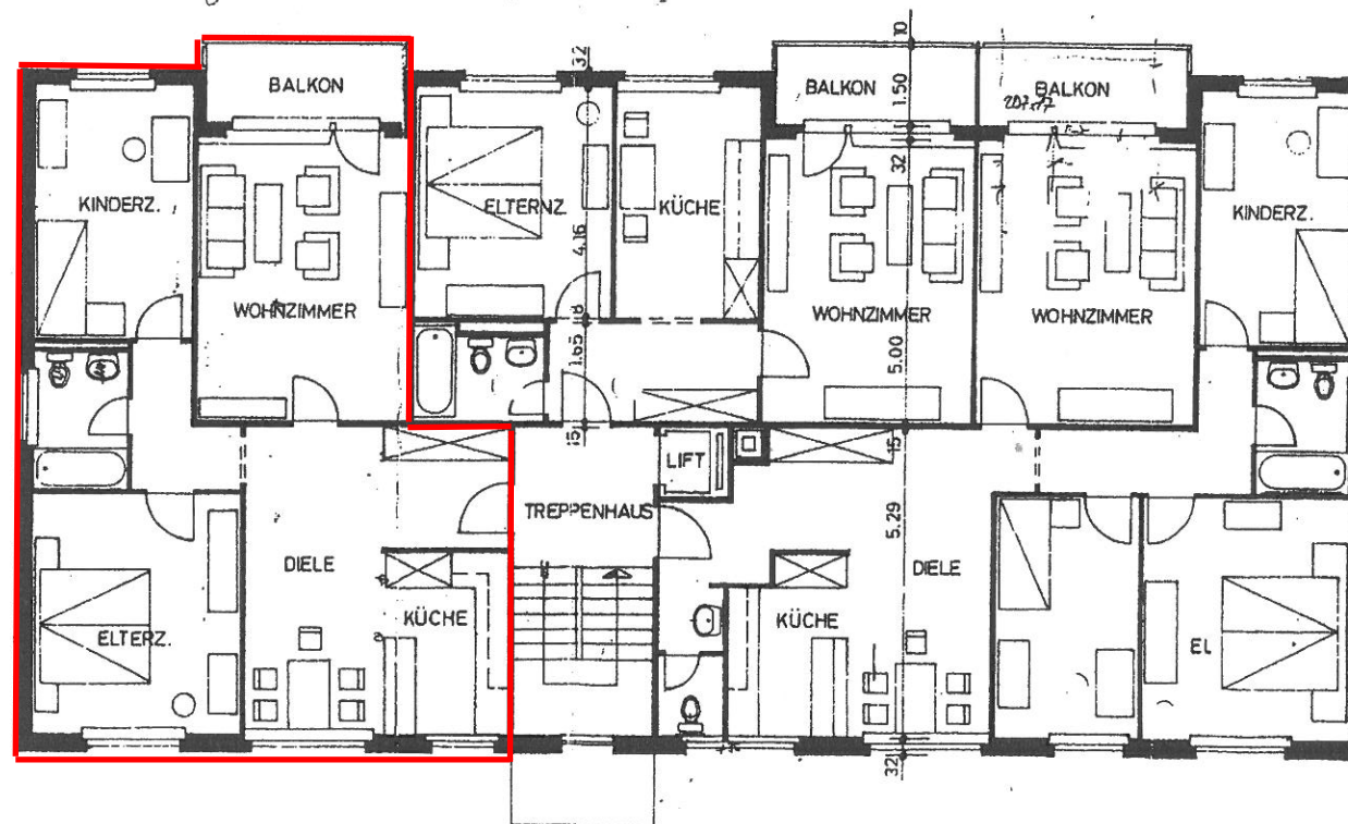
4½-ZIMMERWOHNUNG
